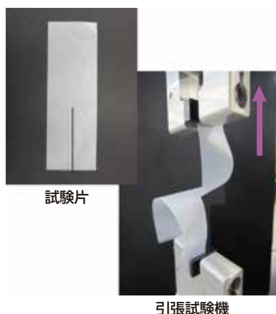
引張試験機
