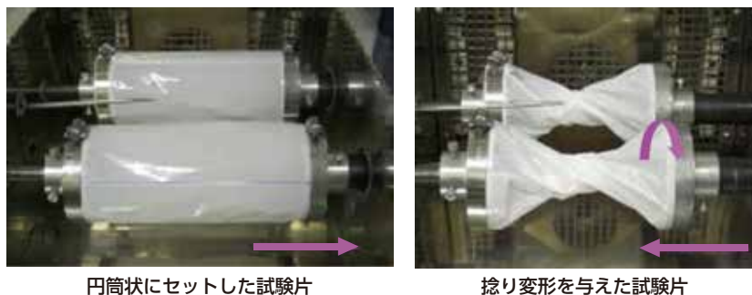
円筒状にセットした試験片
